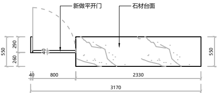
俯视图
