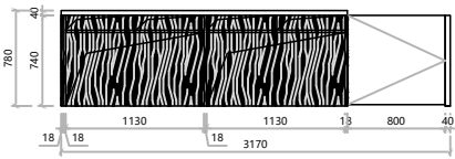
背立面图
