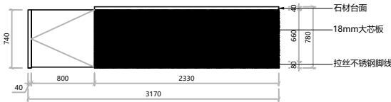
立面图
