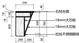
剖面图
